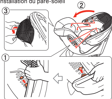
Installation du pare-soleil
